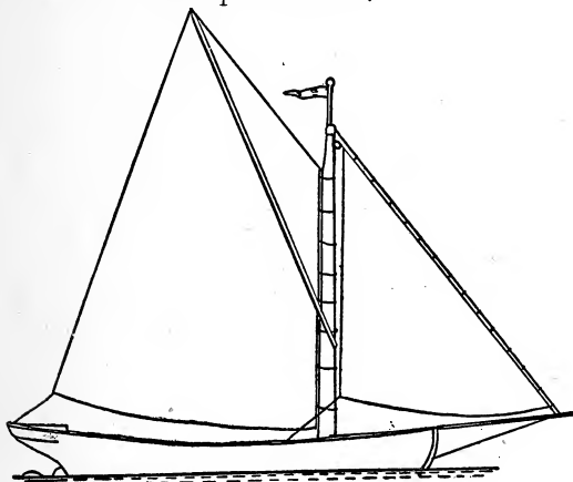
Sprit Rig. Fig. 3.
